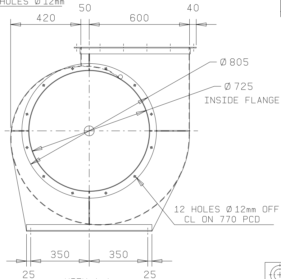
VIEW A-A
